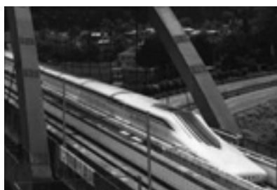
山梨県実験線で地上走行するリニア（JR東海 環境影響評価書より）
